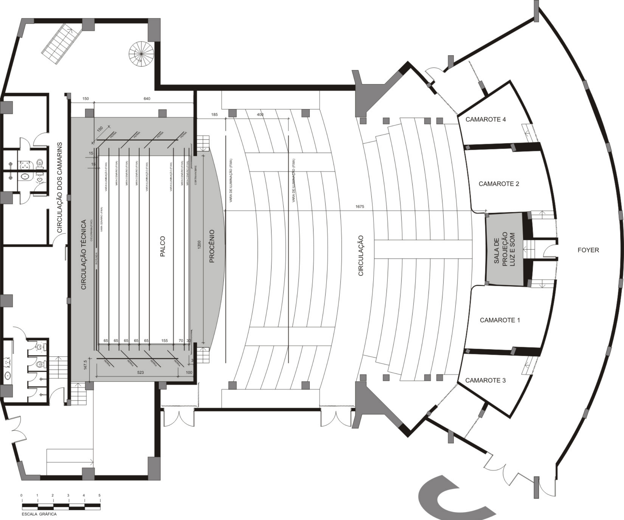
PLANTA PALCO JUAREZ MACHADO
